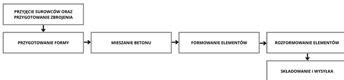
Rysunek 4.1: Uproszczony schemat produkcji płyt stropowych
